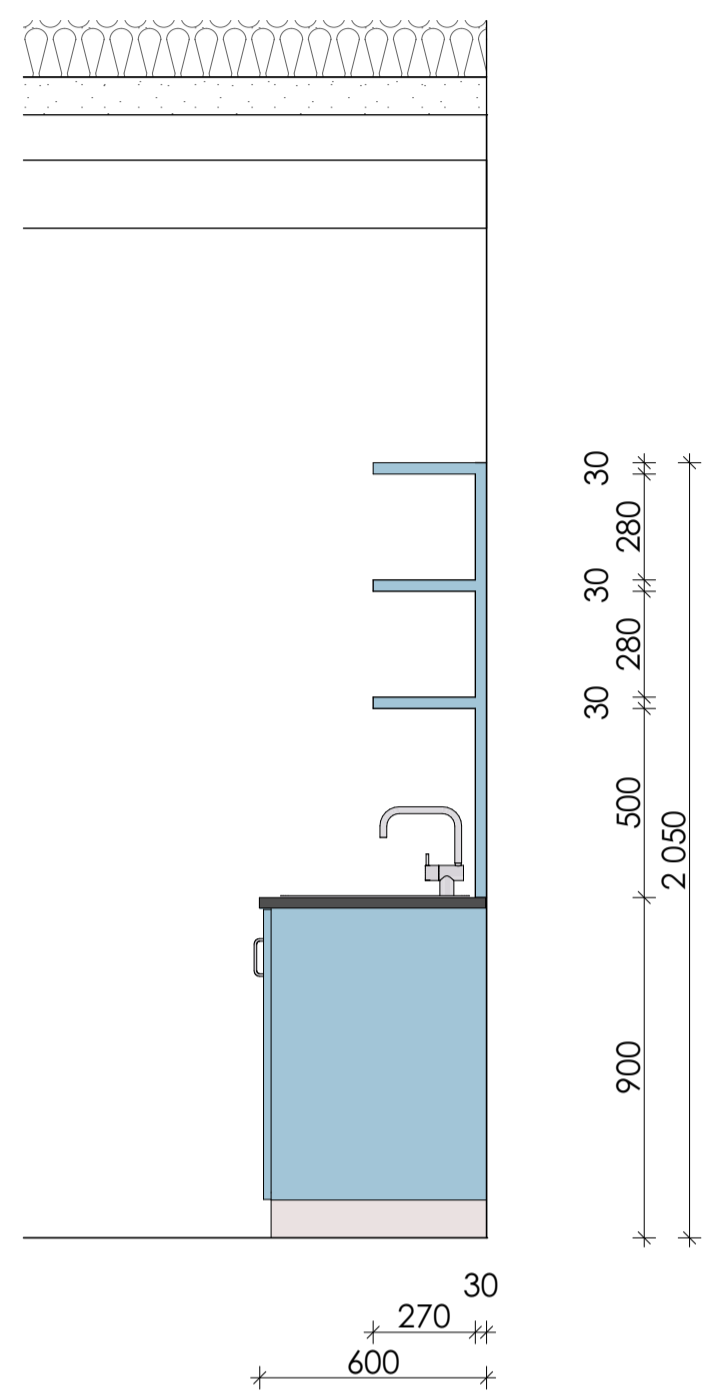
Skjema 02 3.017 kunstrom 1:20
