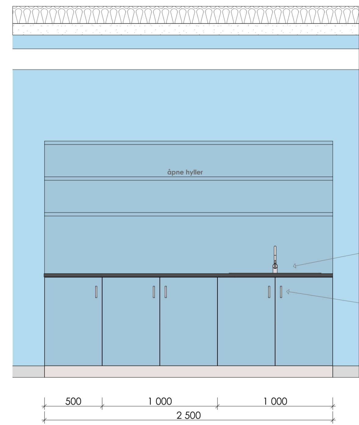
Skjema 01 3.017 kunstrom 1:20
