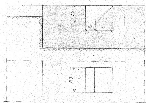
Detalj I M=1:10
