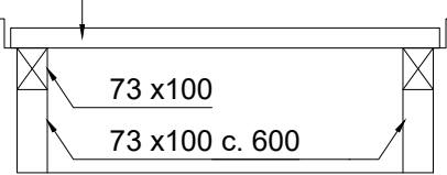
Snitt, 1:20
