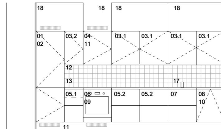
Oppriss - kjøk. personal
