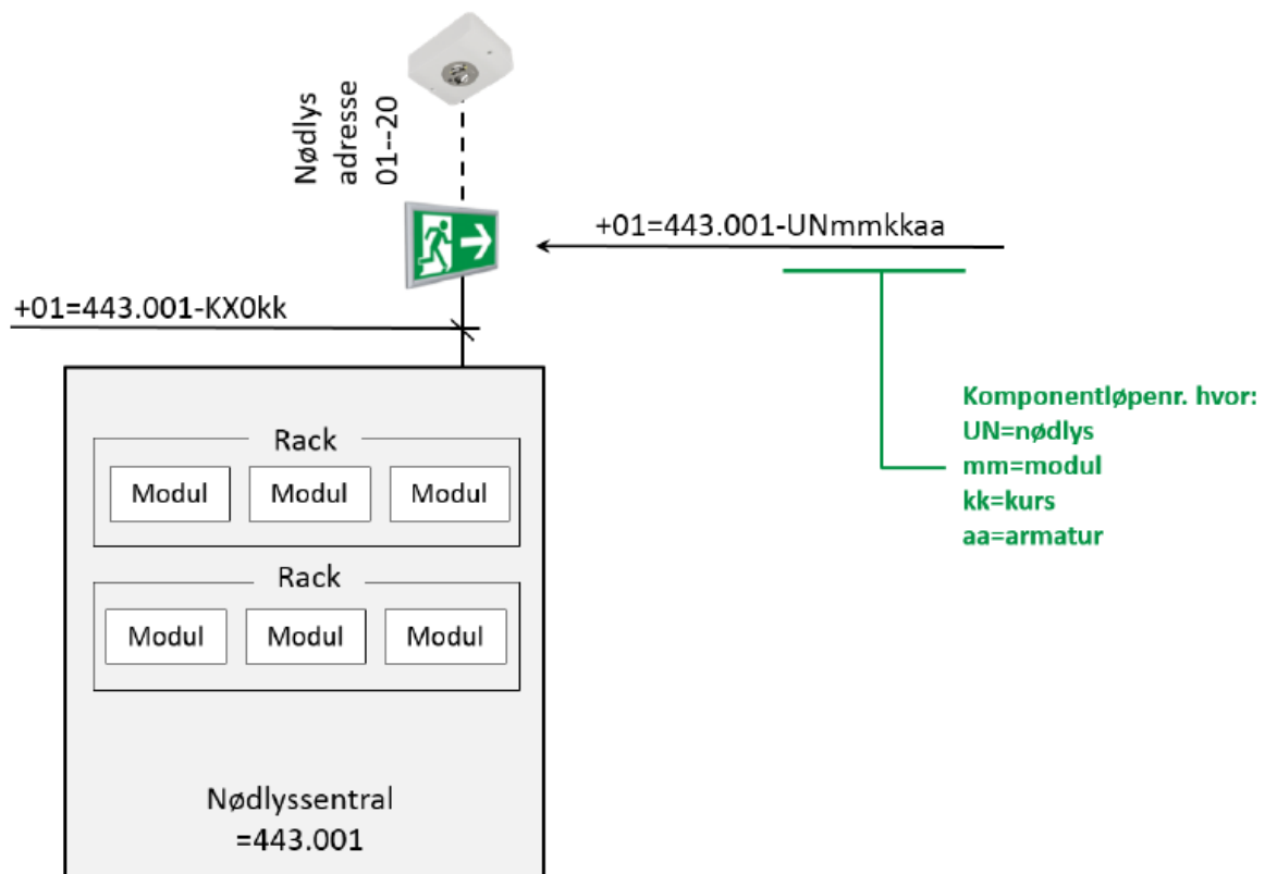
Figur 6-1 Topologiskjema for nødlysanlegg
