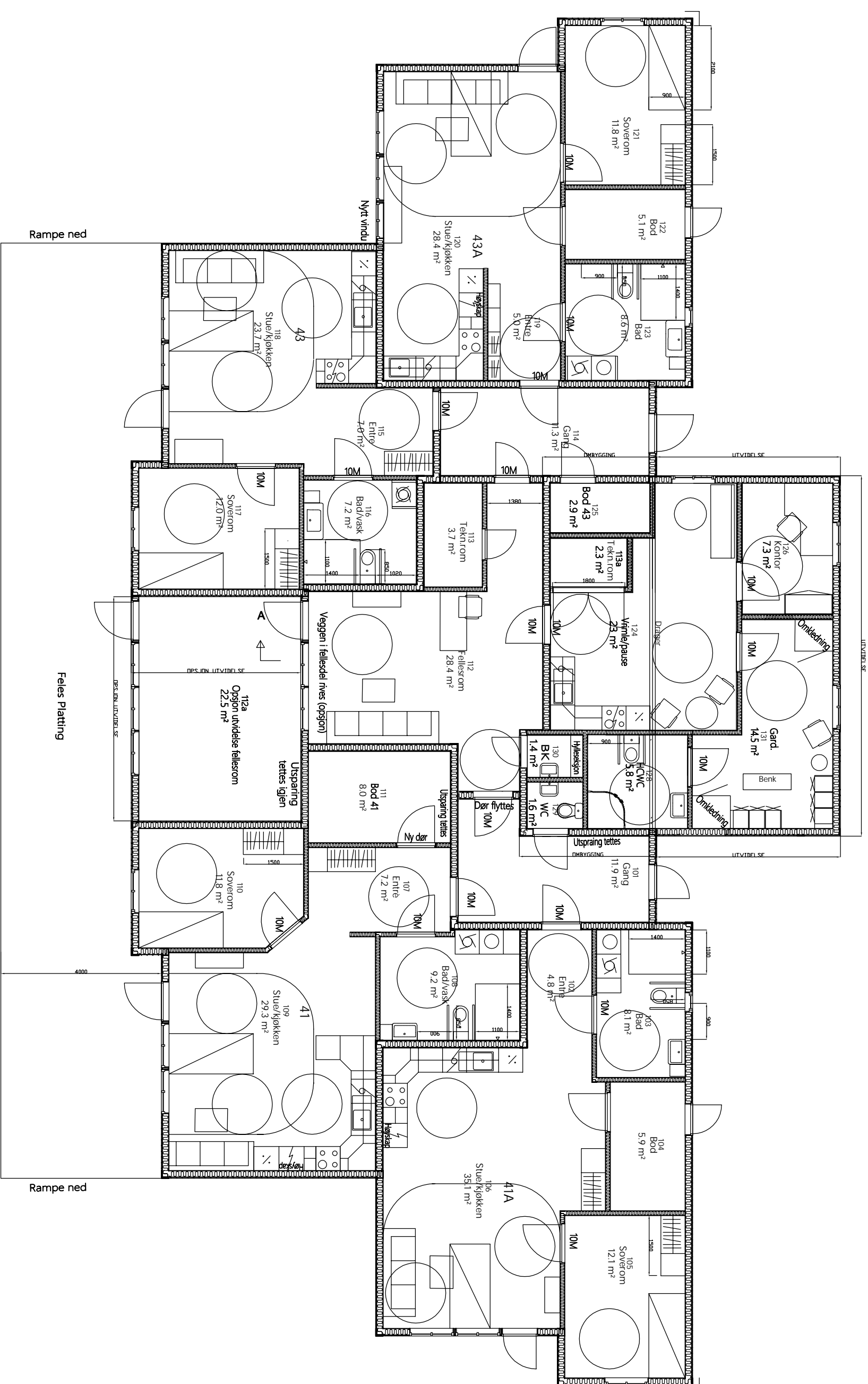
Plan 1. etg
