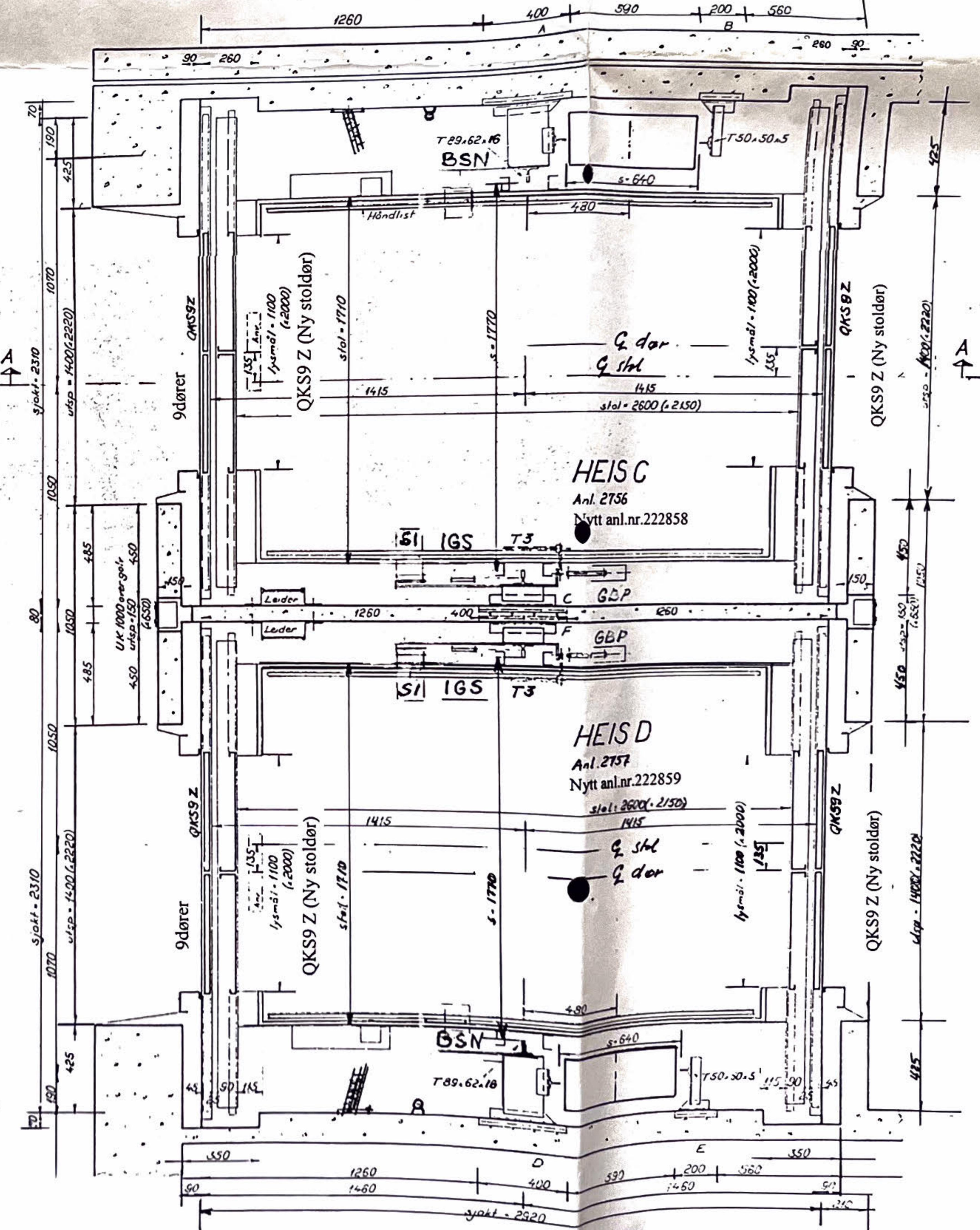
GRUNNRIS AV SJAKTER OG STOLER 1:20
