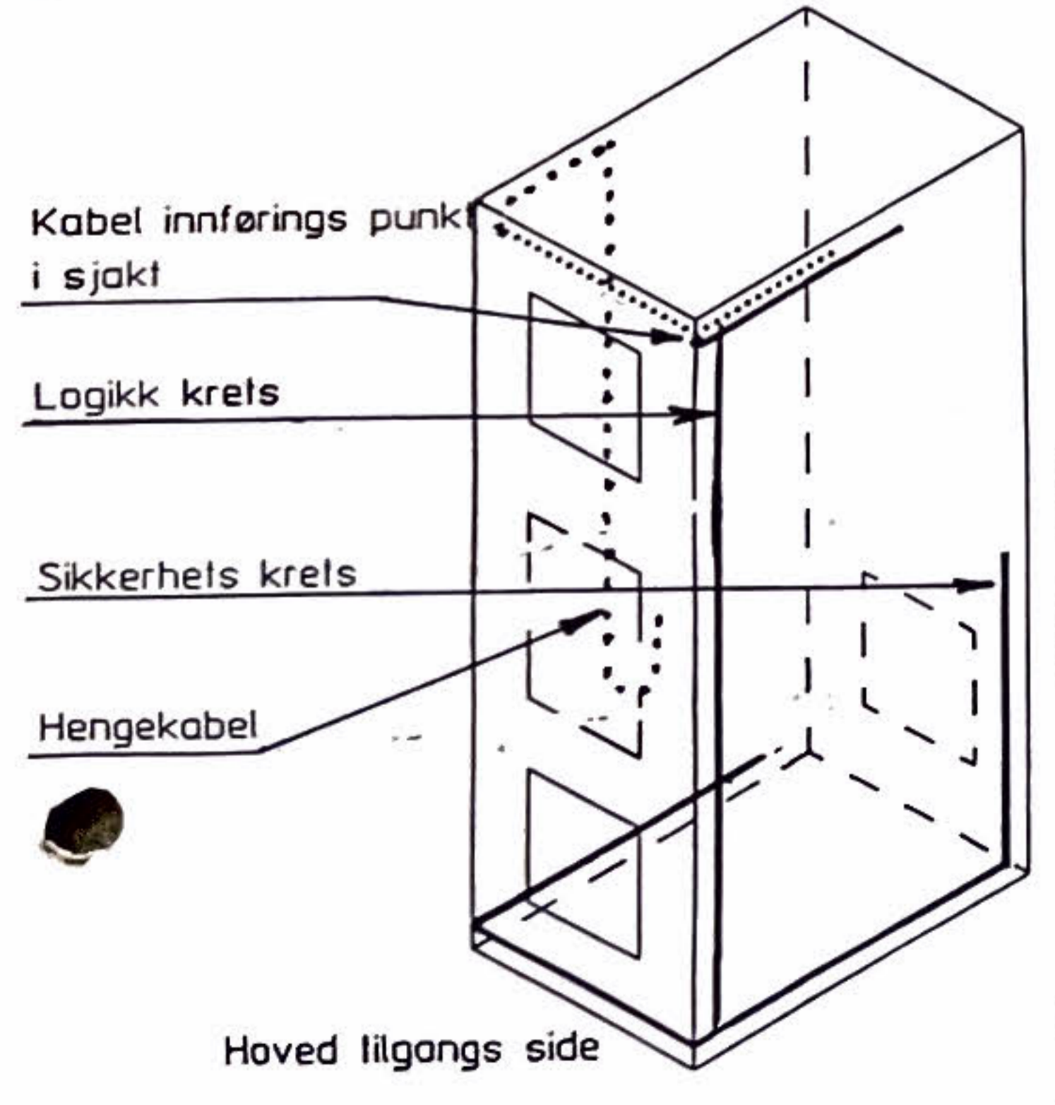
Kabelarrangement Anl.222858.Heis C.
