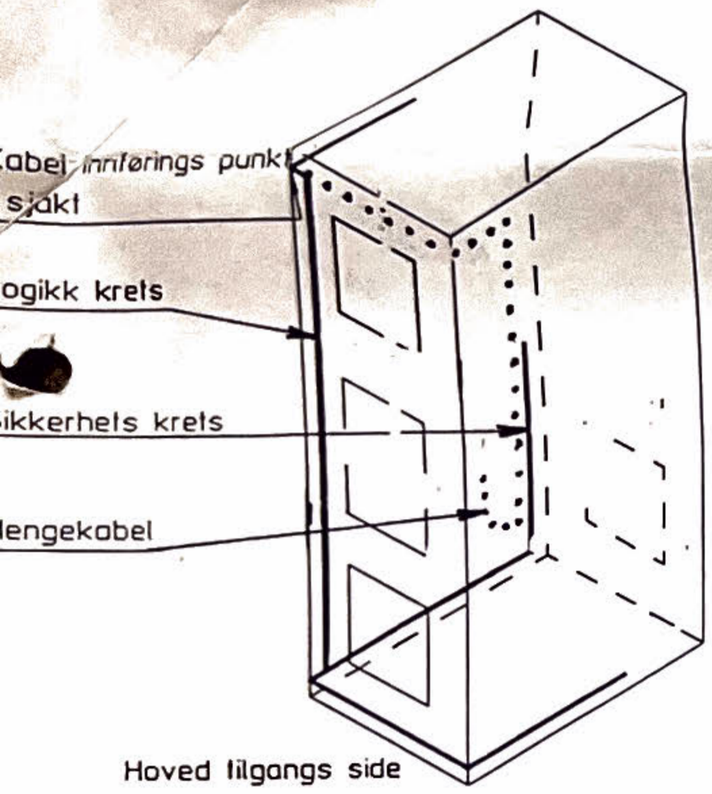
Kabelarrangement Anl.222859.Heis D.
