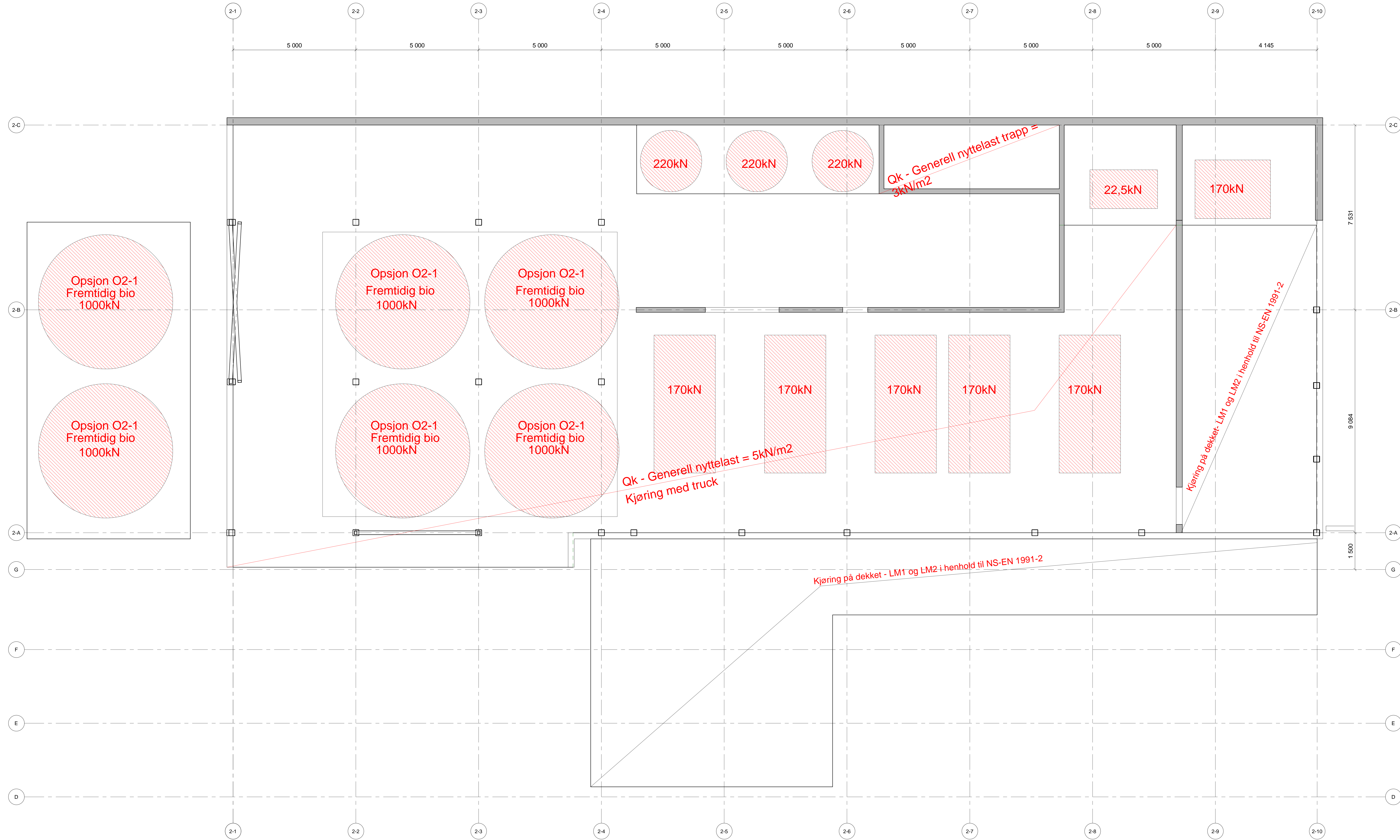
LASTPLAN - GOLVPLAN 1 : 50
