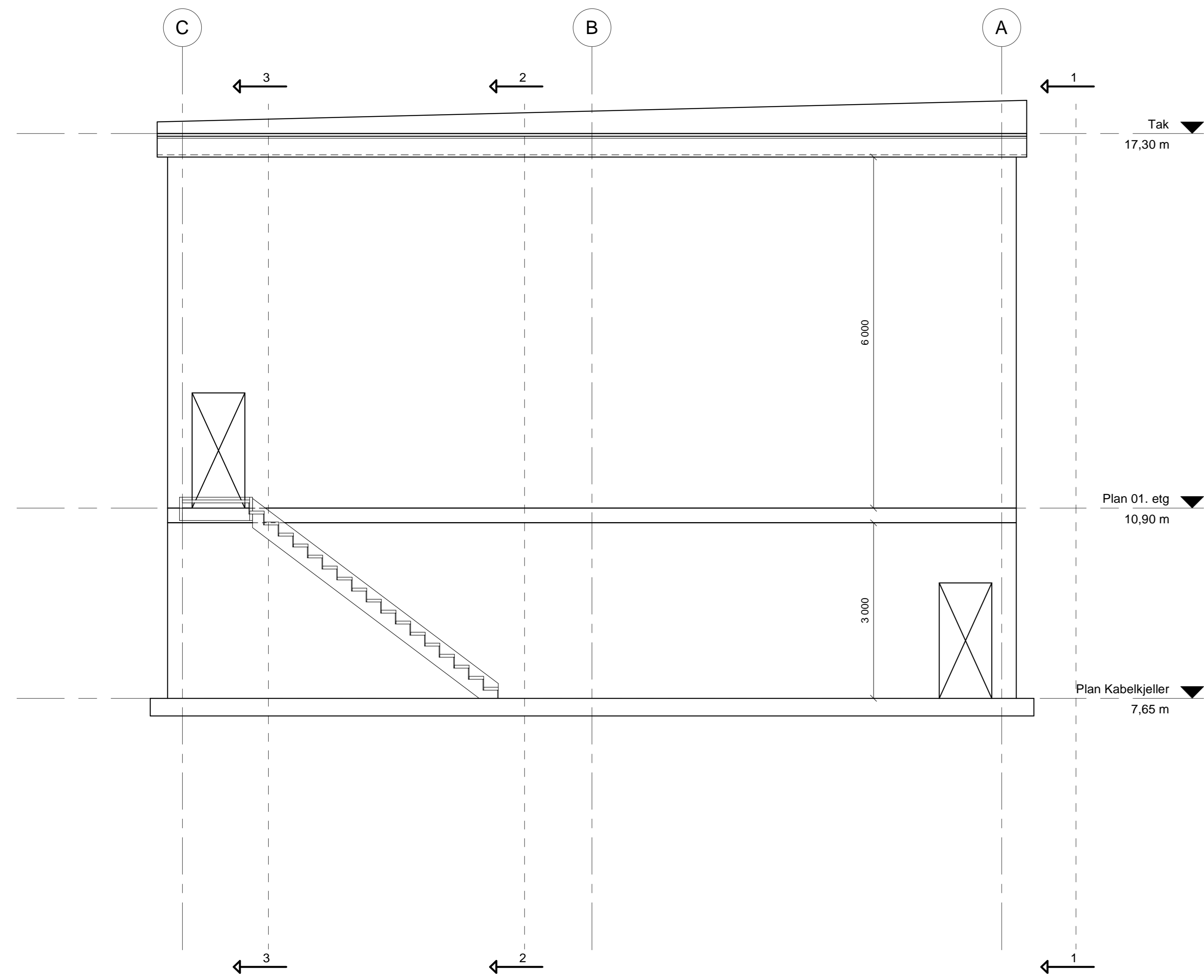
SNITT 4 1 : 50
