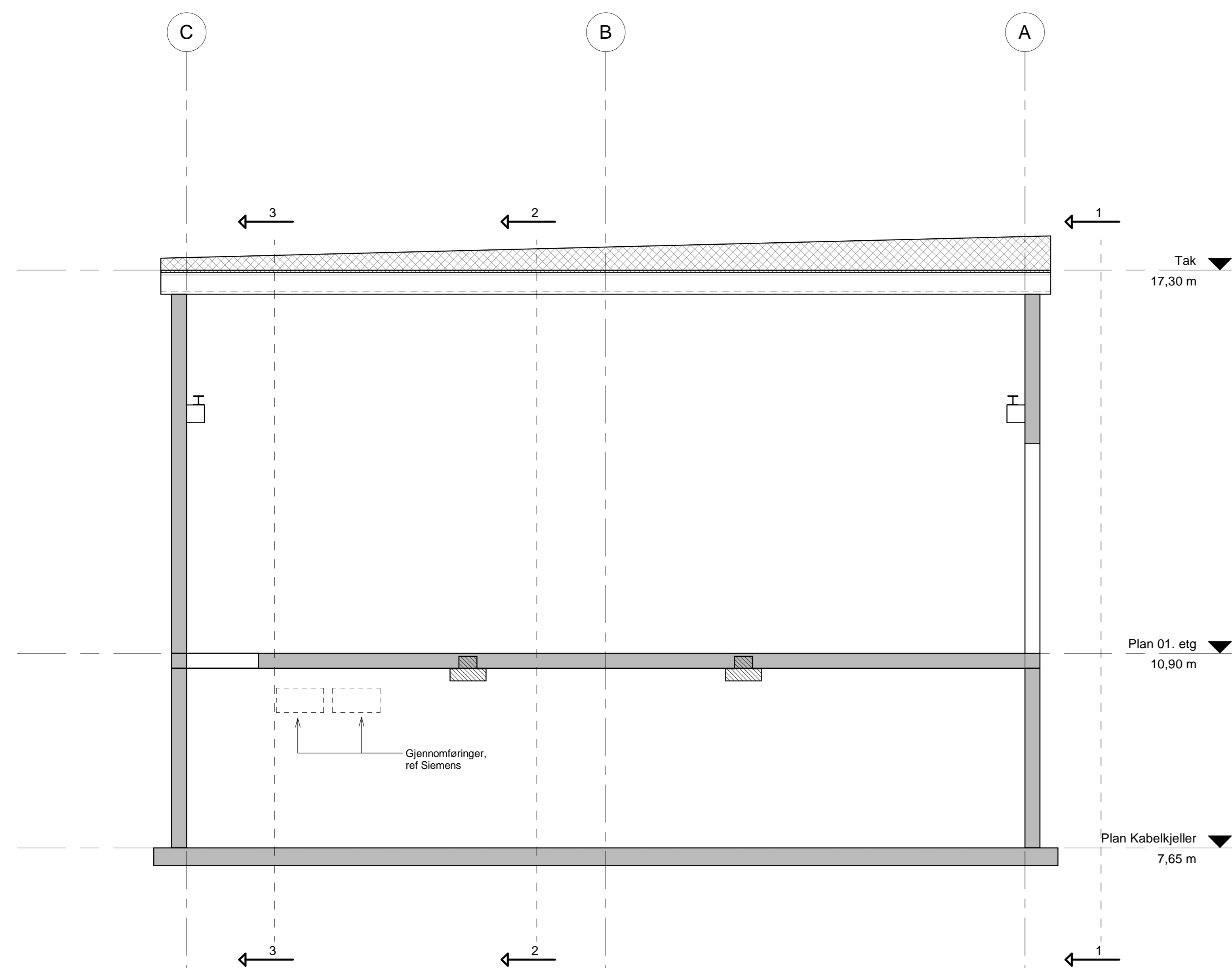
SNITT 6 1 : 50
