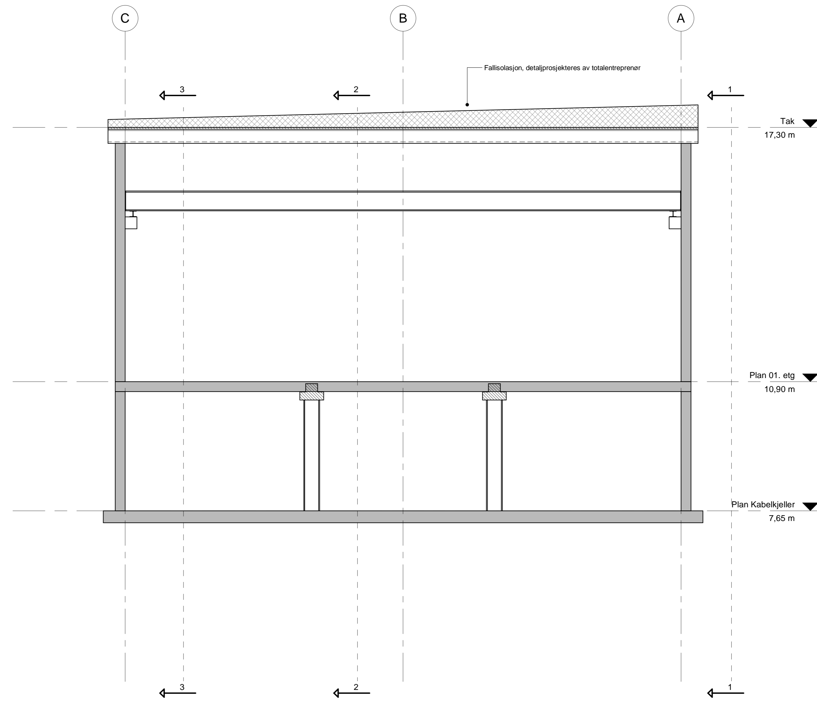
SNITT 5 1 : 50
