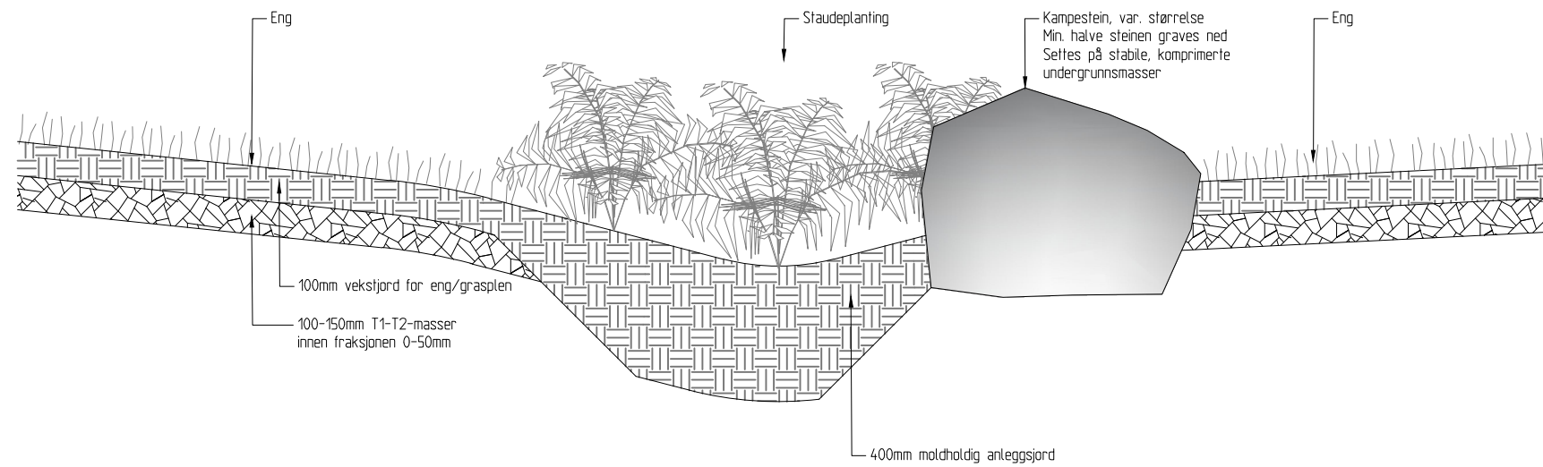
KAMPESTEIN OG STAUDEPLANTING I OVERVANNSGRØFT SNITT
