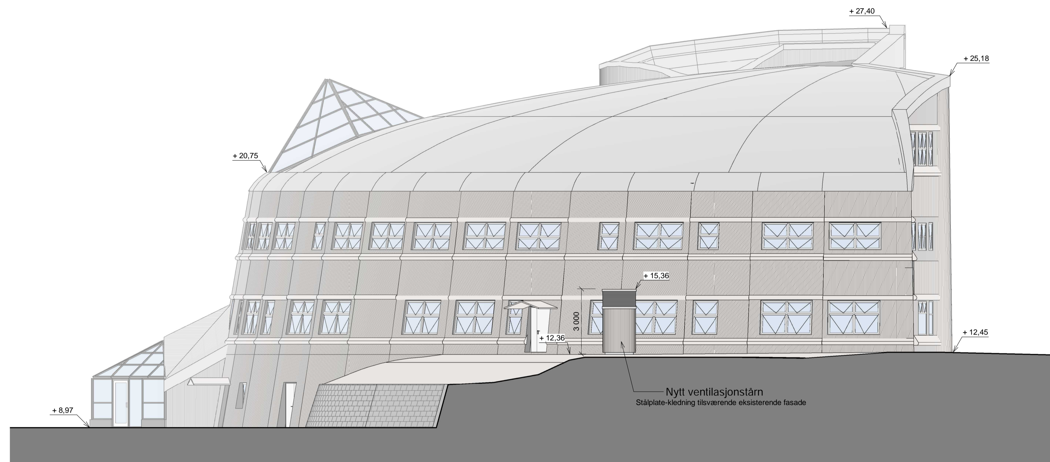
Fasade nord - øst 1 : 100
