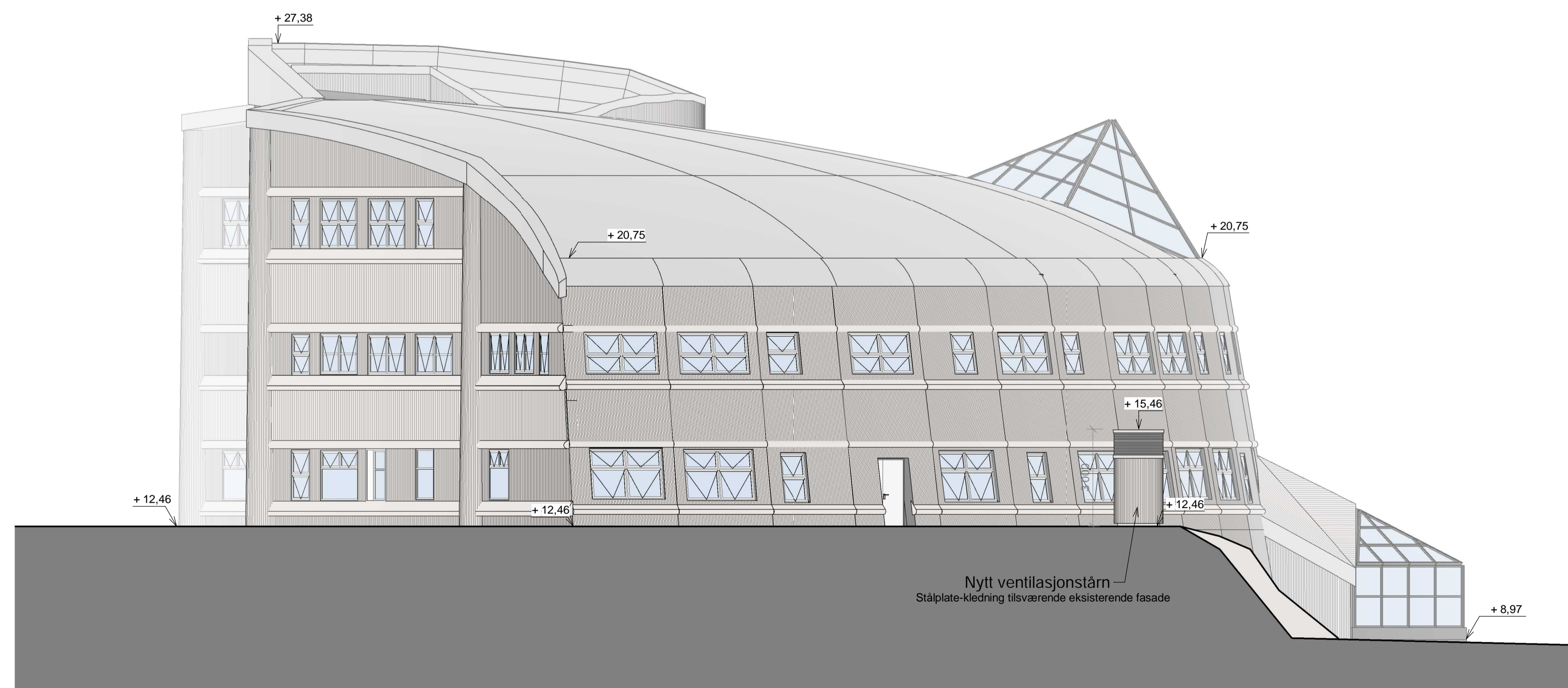
Fasade sør - vest 1 : 100
