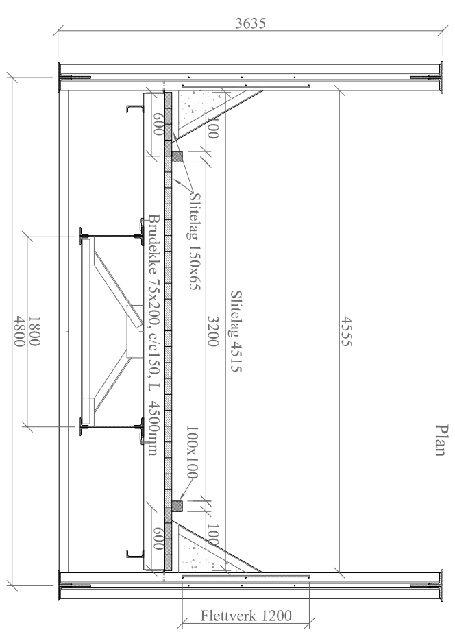
Snitt A-A
