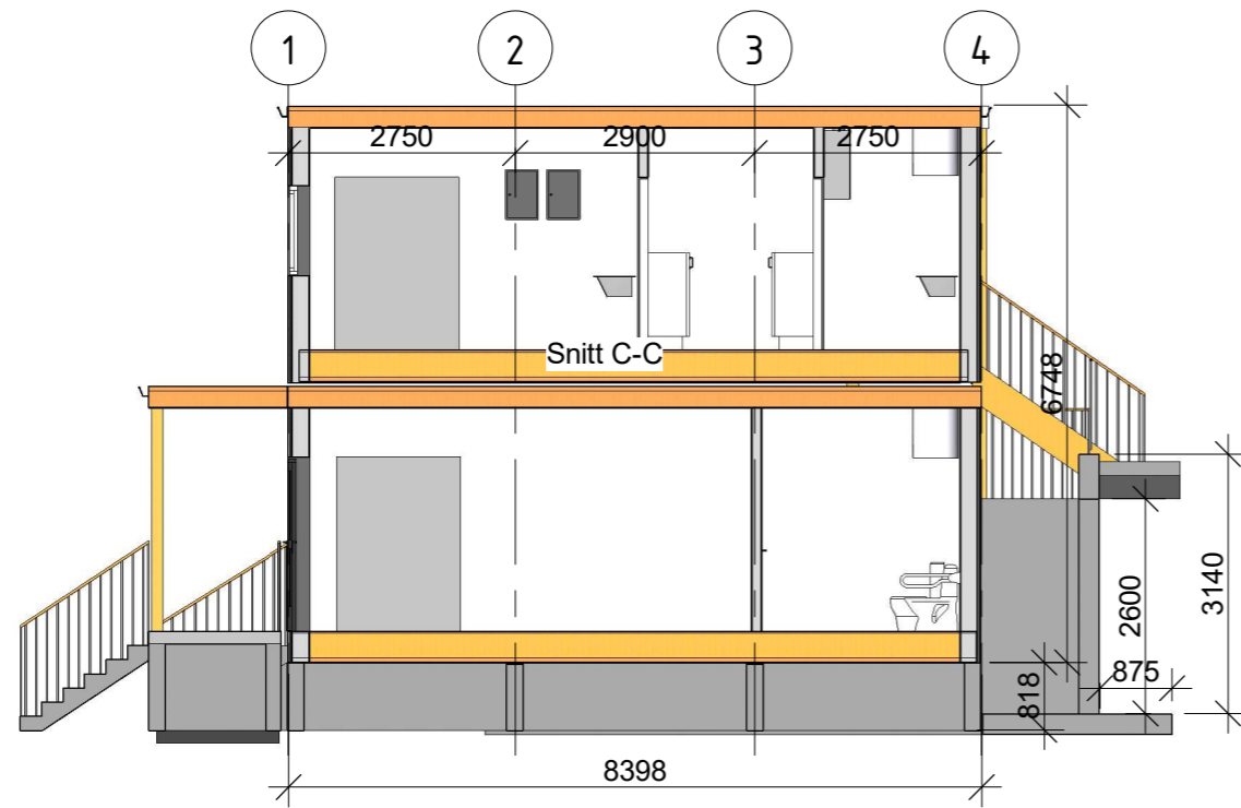
Snitt C - C 1 : 100
