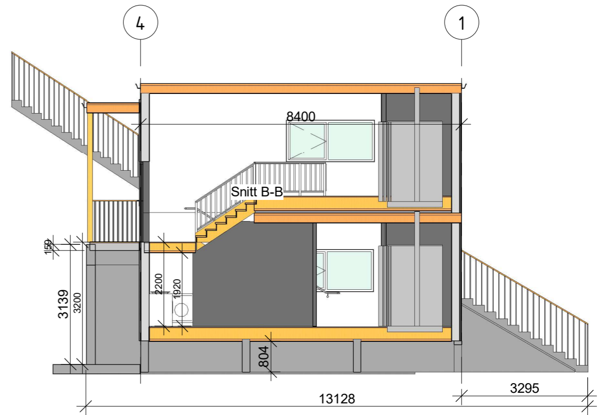
Snitt B - B 1 : 100
