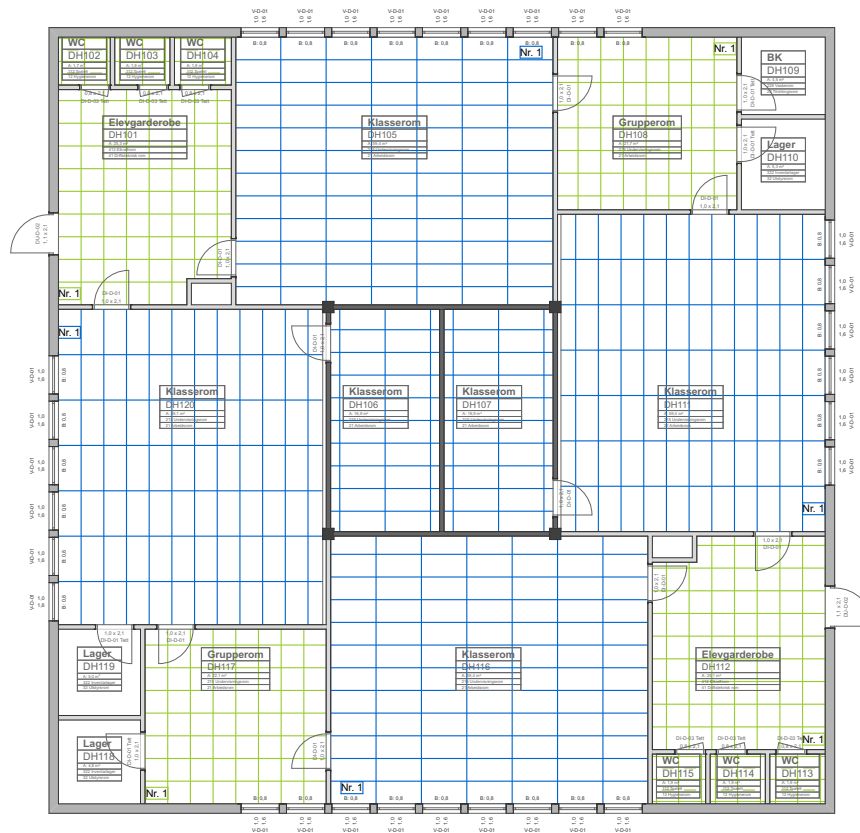
Bygg D - 1. Etasje
